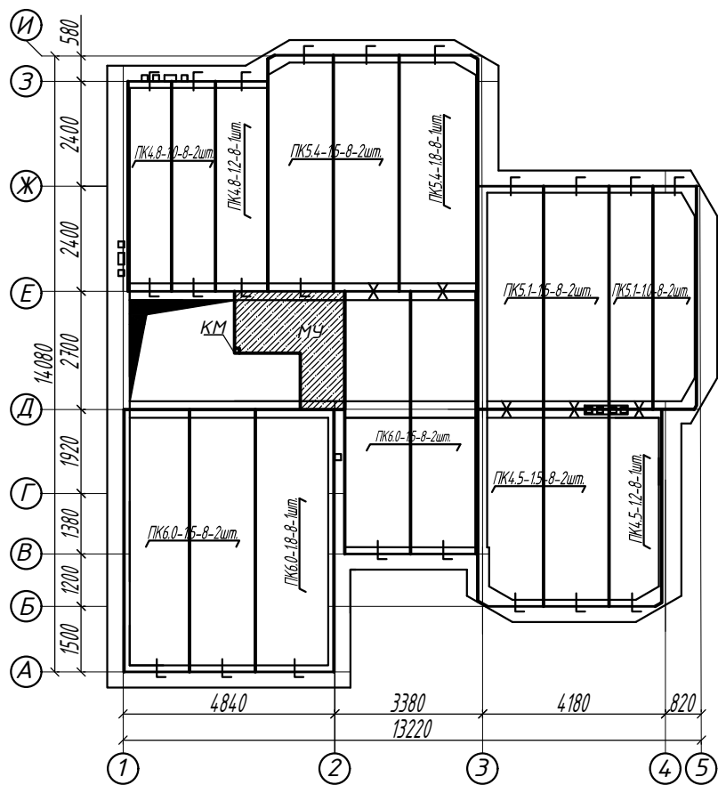
План плит перекрытия на отметке +2.900
