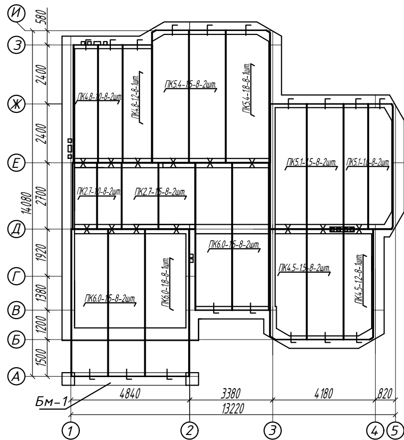
План плит перекрытий на отметке +6.200
